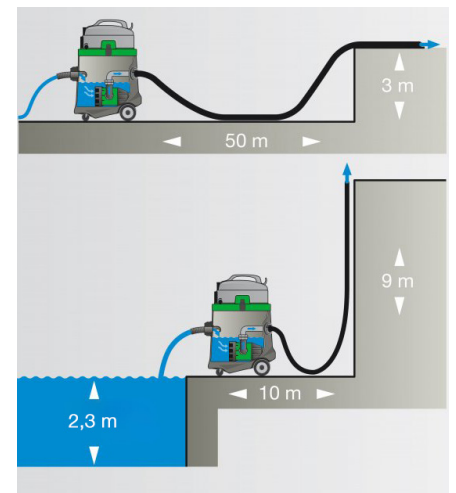
Schema zuig- en pompbereik
