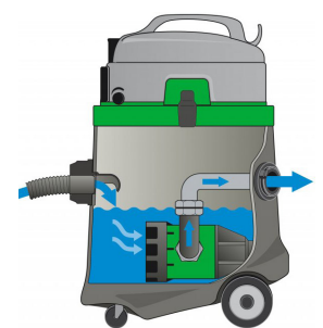
Functionieschema
